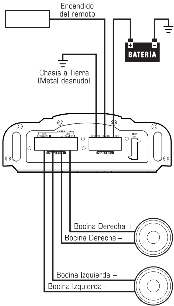
Figura 3 Conexiones para la potencia y las bocinas
